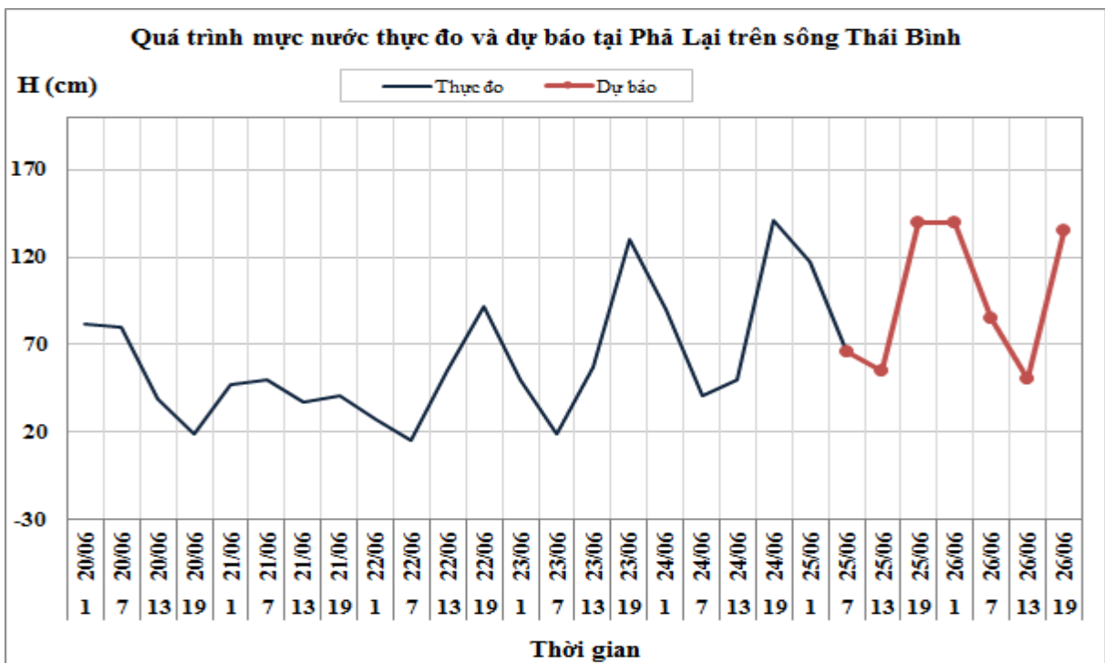
Hình 2: Quá trình mực nước thực đo và dự báo tại trạm Phả Lại trên sông Thái Bình
